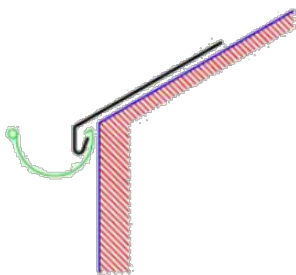
Abbildung 3: Einlaufblech
