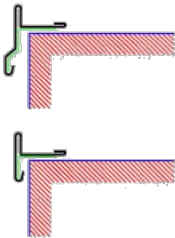
Abbildung 9: Giebeleinfassung
