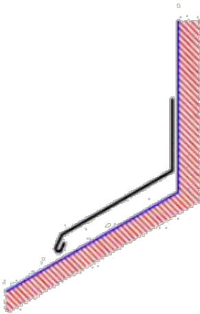
Abbildung 15: Brustblech
