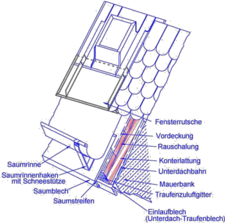
Abbildung 53: Fensterrutsche
