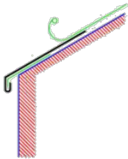
Abbildung 1: Saumblech
